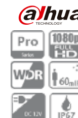
DH-HAC-HFW2231R-Z6 CÁMARA IP HDCVI TUBO EXTERIOR 2.1MP | 2.7-13.5mm | IR:60m | IP67 | WDR
